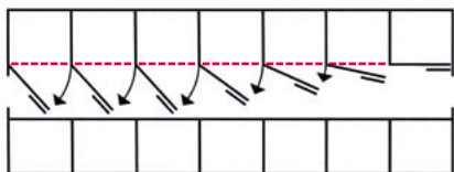
Stalschema met volledig wegdraaibare voorwanden
